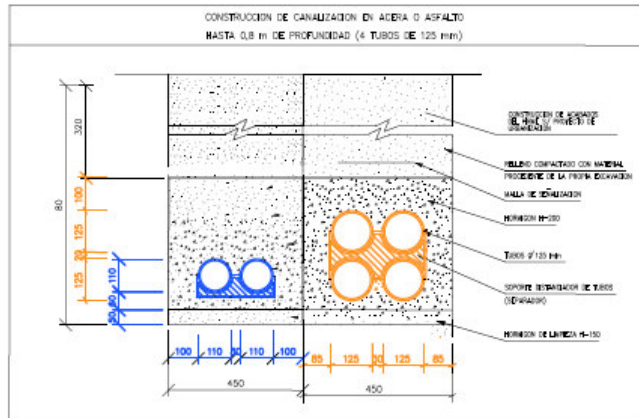
CANALIZACION 2T 110mm. TELEFONICA + 4T 125mm. EUSKALTEL
