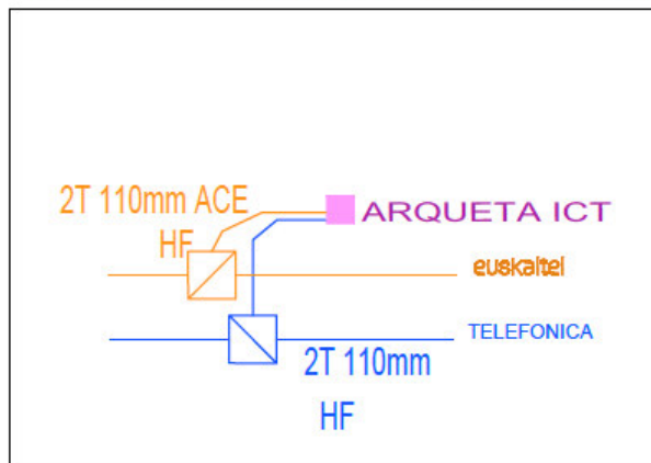
DETALLE ACOMETIDA A CADA ICT DESDE TELEFONICA Y EUSKALTEL
