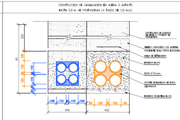
CANALIZACION 4T 110mm. TELEFONICA + 4T 125mm. EUSKALTEL
