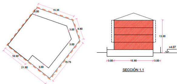
SEMISOTANO/SOTANO (Garajes)
