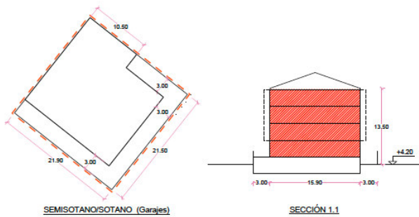
SEMISOTANO/SOTANO (Garajes)
