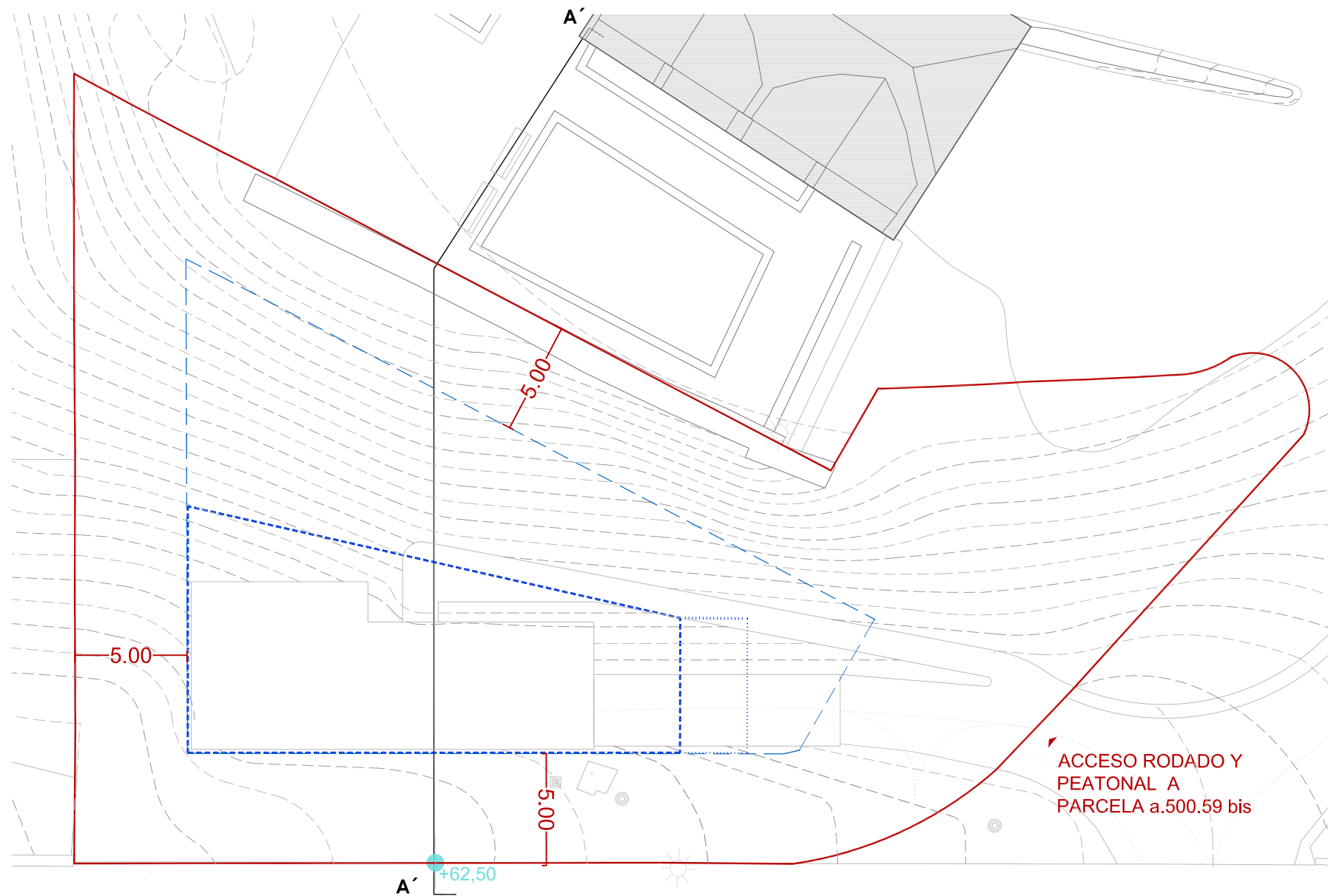
PLANTA
