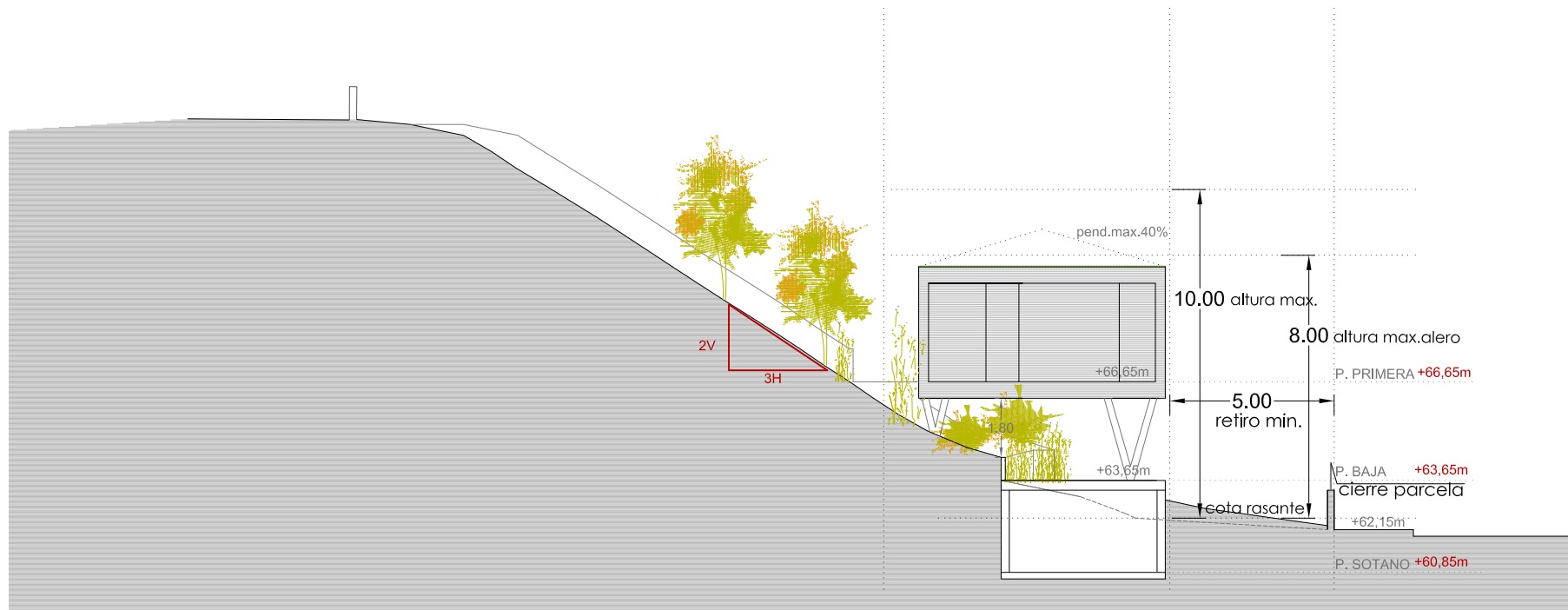
SECCIÓN B-B'
