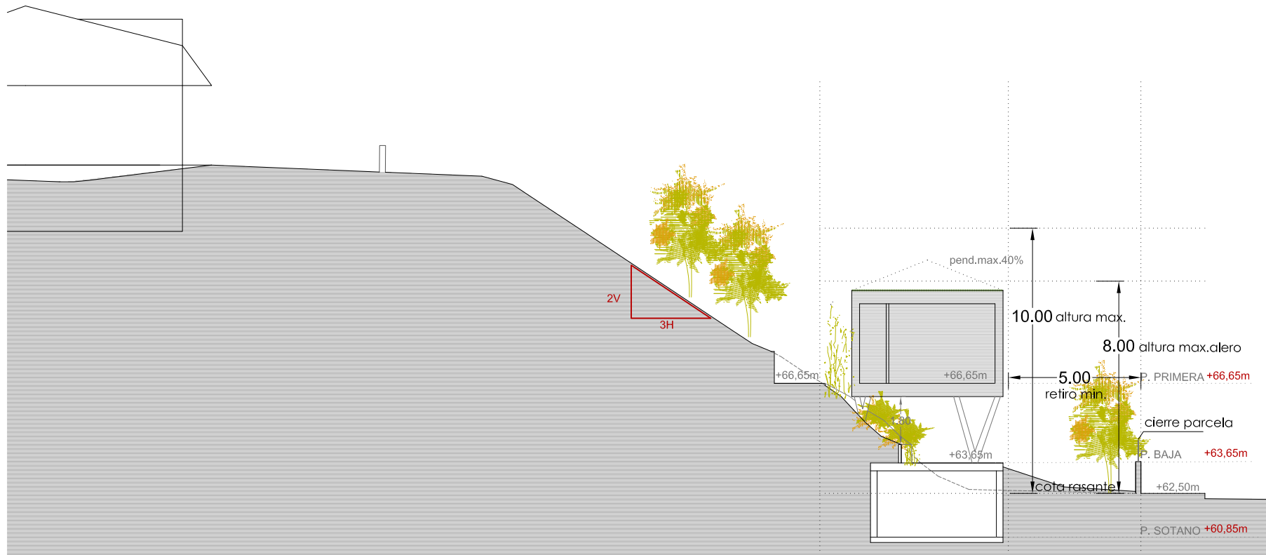
SECCIÓN A-A'
