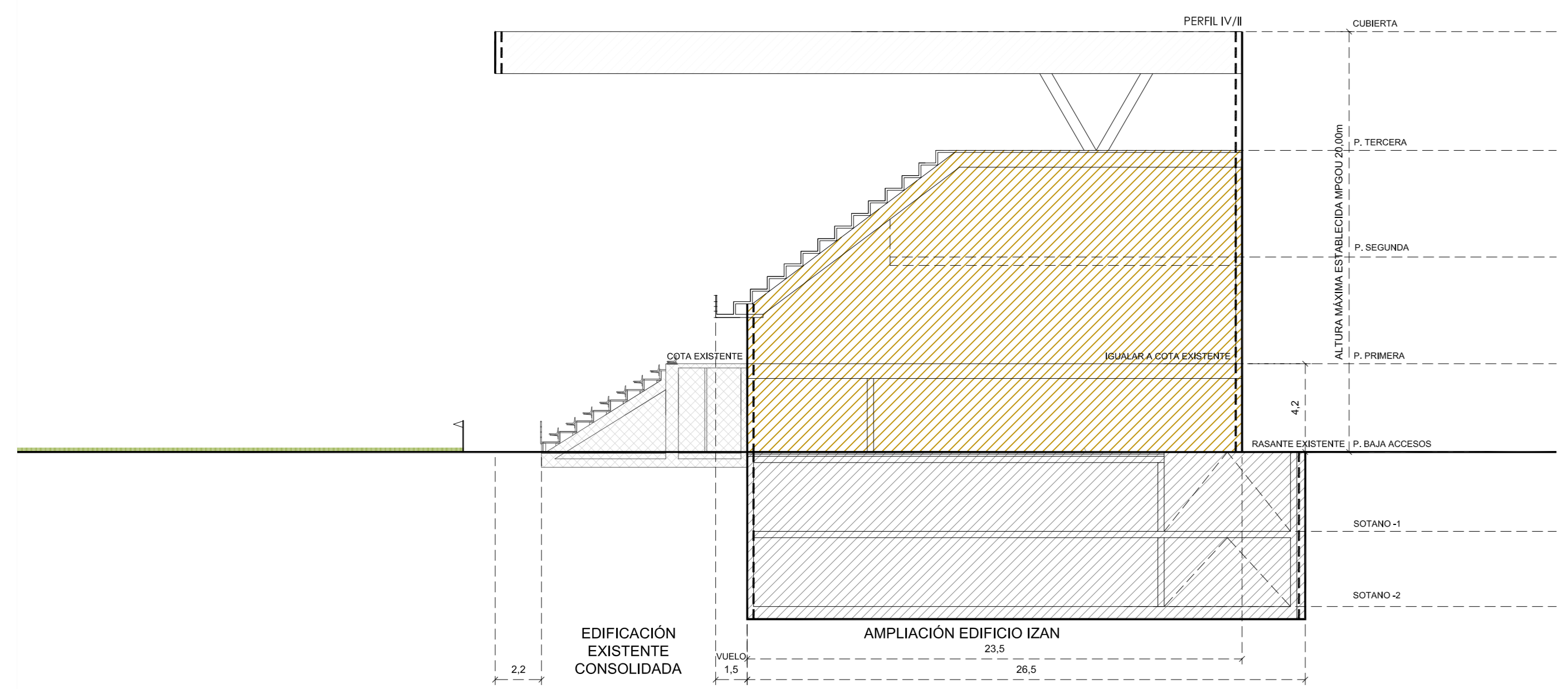
SECCIÓN ENVOLVENTE MÁXIMA AA
