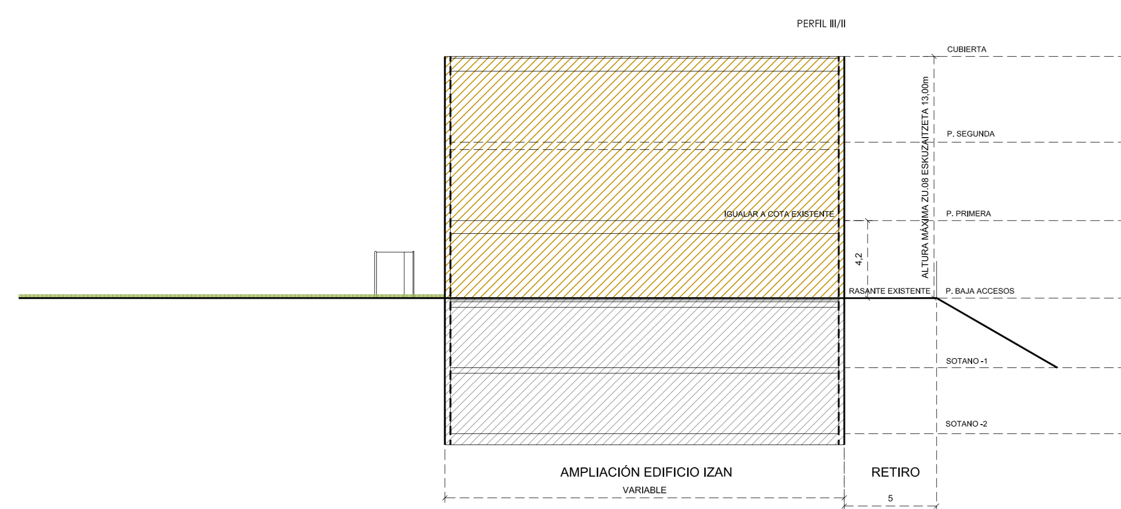
SECCIÓN ENVOLVENTE MÁXIMA BB
