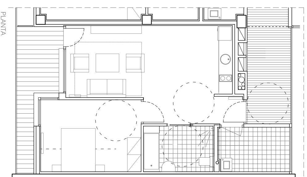
APARTAMENTO ADAPTADO TIPO 3 - 58 m 2
