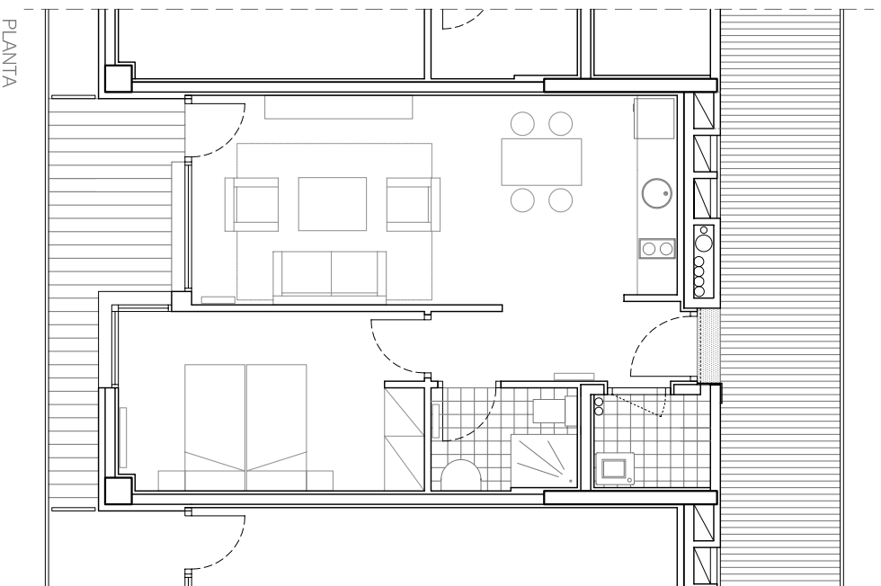
APARTAMENTO TIPO 1 - 50 m 2
