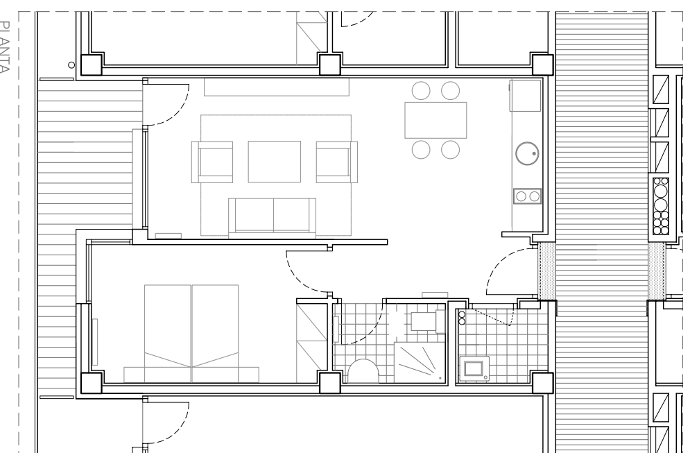
APARTAMENTO TIPO 2 - 51 m 2
