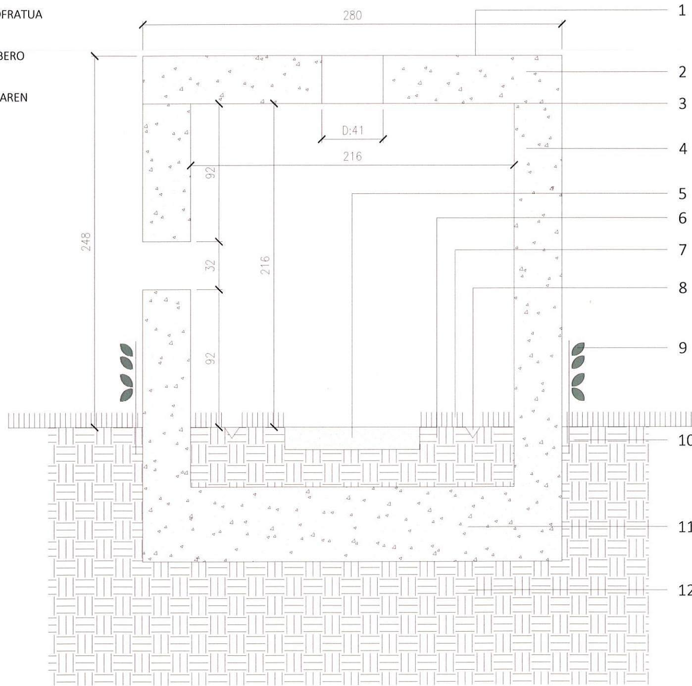
ZEHARKAKO EBAKIDURA E:1/25
