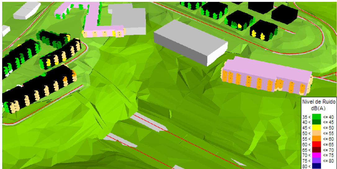
Niveles en fachada sin soluciones. Periodo noche
