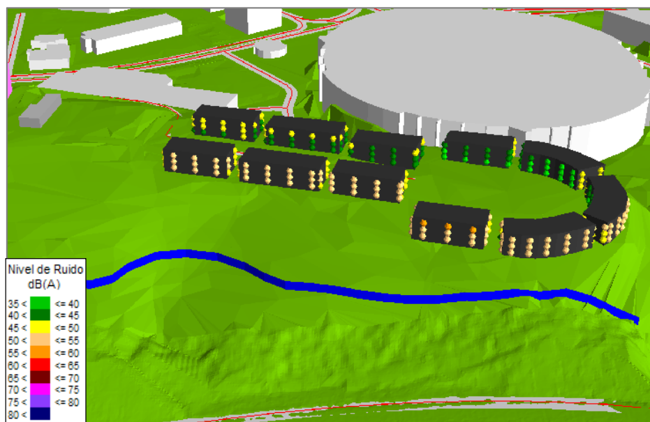
Nivel de ruido en fachada 3D con solución. Periodo noche
