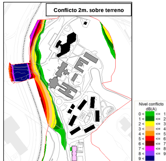
Exceso de dB(A) por encima de los OCA establecidos a 2m y en fachadas. Tráfico de carreteras
