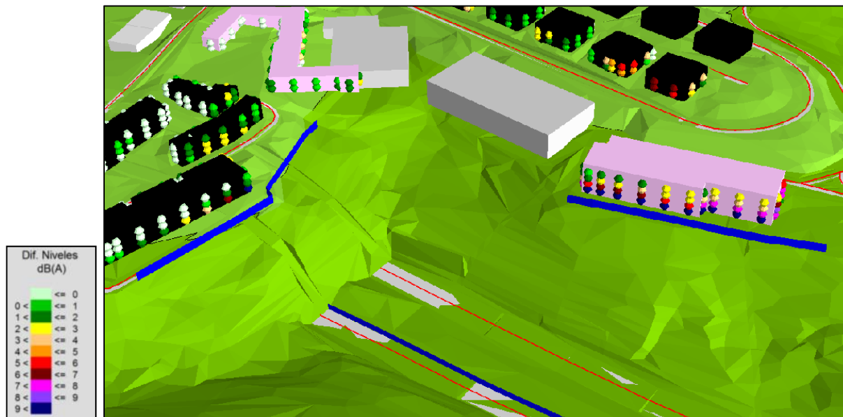
Beneficio acústico generado por la pantalla (OCA: L_n=55 dB(A))
