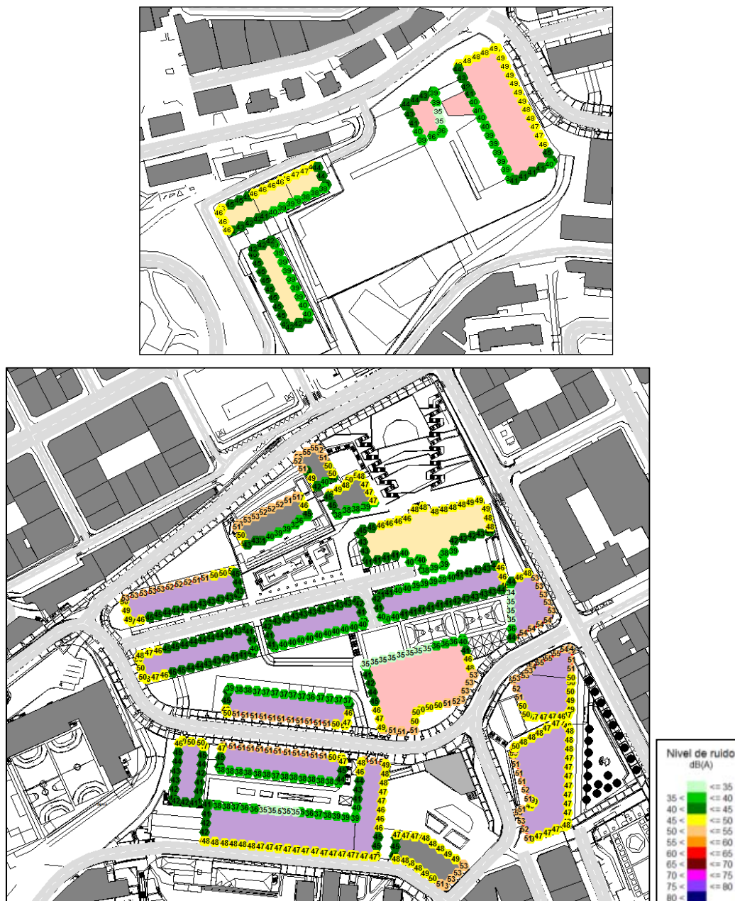
Mapa de fachadas 2D del escenario futuro incluyendo la reducción de velocidad. Periodo noche
