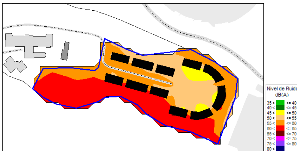
Nivel de ruido obtenido a 2m. de altura. Periodo día
