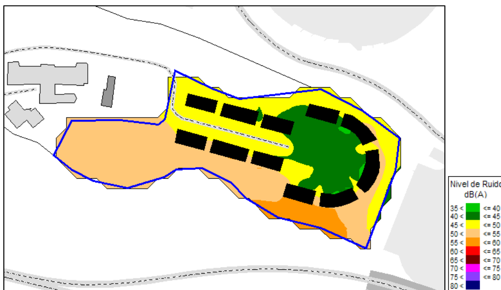
Nivel de ruido obtenido a 2m. de altura. Periodo noche
