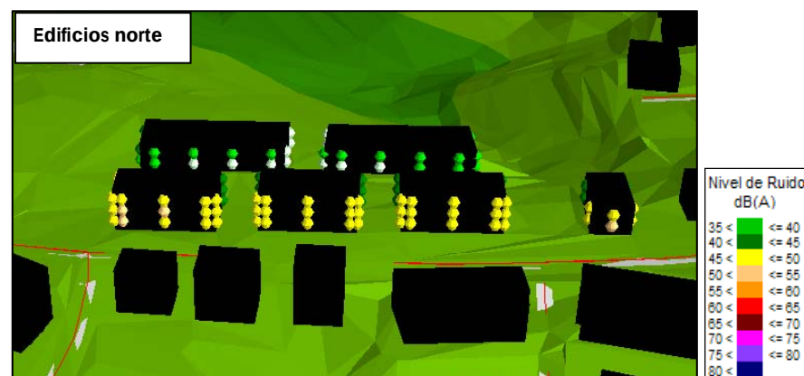
Nivel de ruido en fachada. Periodo noche
