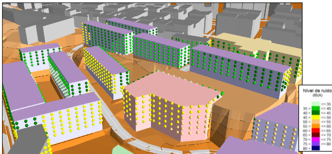
Mapas de fachadas 3D del escenario futuro incluyendo la reducción de velocidad. Periodo noche
