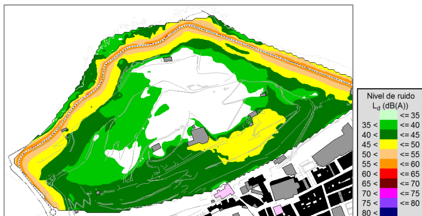
Nivel de ruido periodo día.
