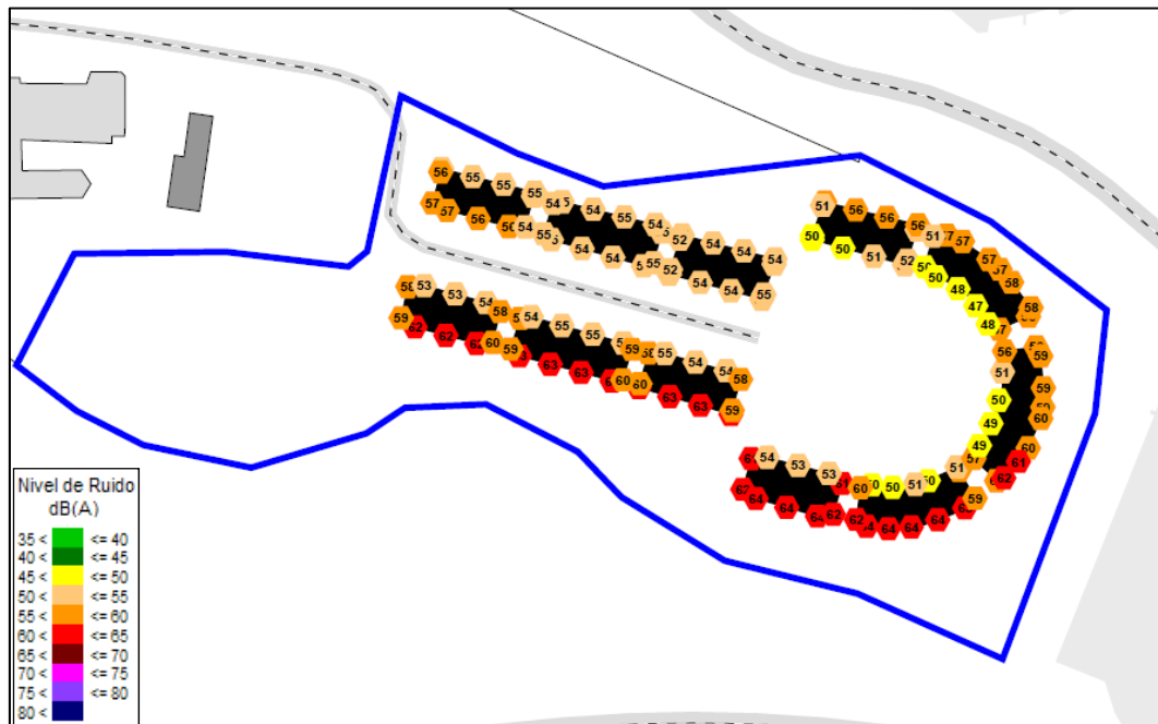
Nivel de ruido en fachada. Periodo día
