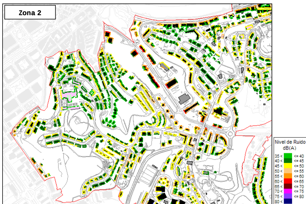
Mapas de fachadas a todas las alturas (se muestra el nivel de ruido a la altura más afectada)
