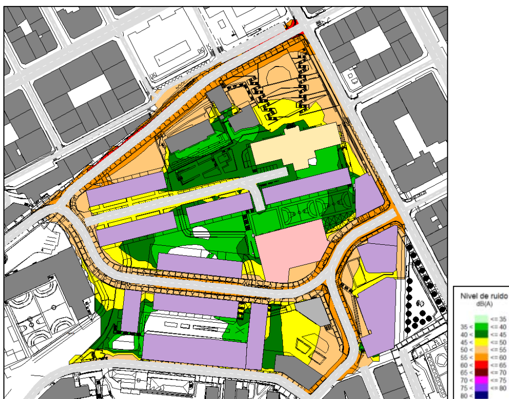
Mapa de ruido 2m. del escenario futuro incluyendo la reducción de velocidad. Periodo noche
