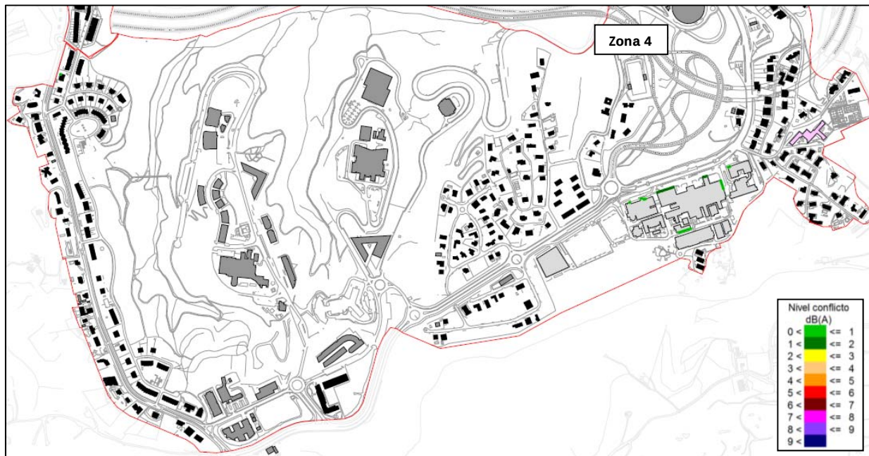
Exceso de dB(A) por encima de los OCA establecidos en fachadas. Tráfico de calles
