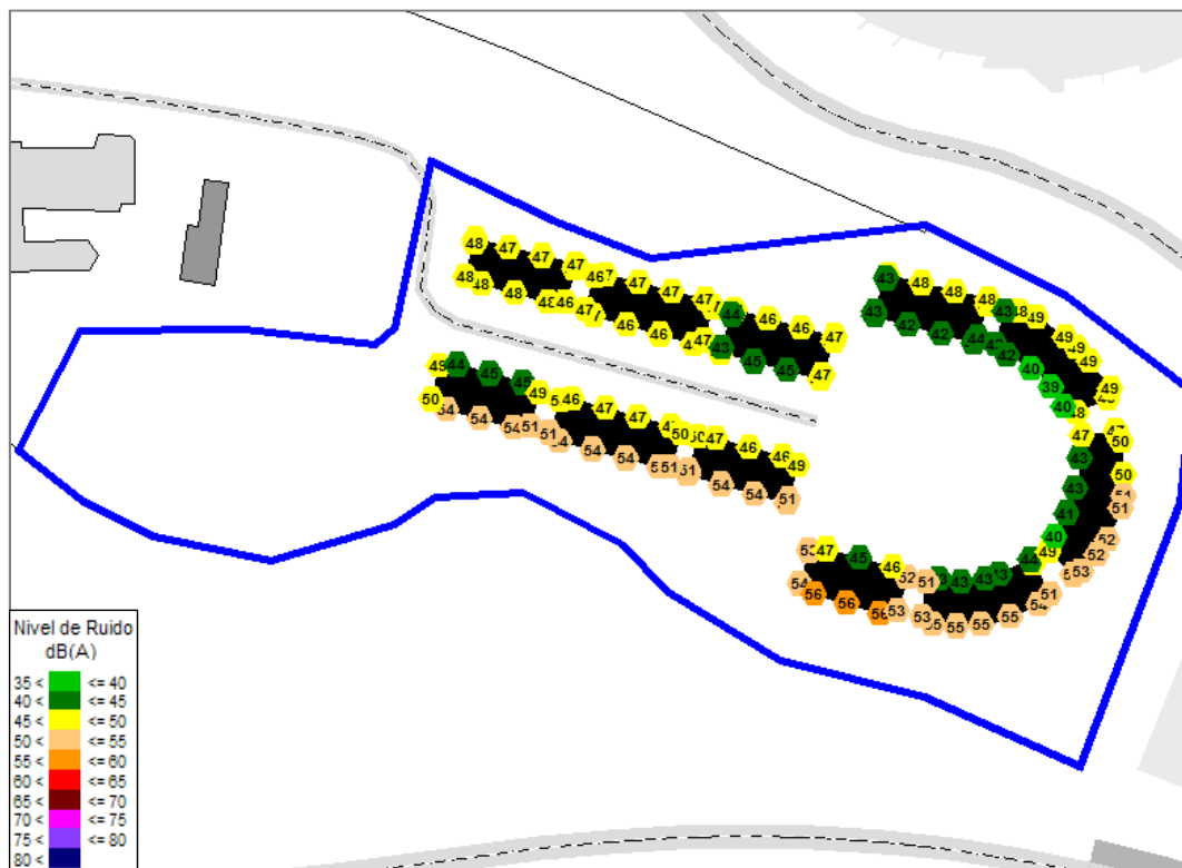
Nivel de ruido en fachada con solución. Periodo noche
