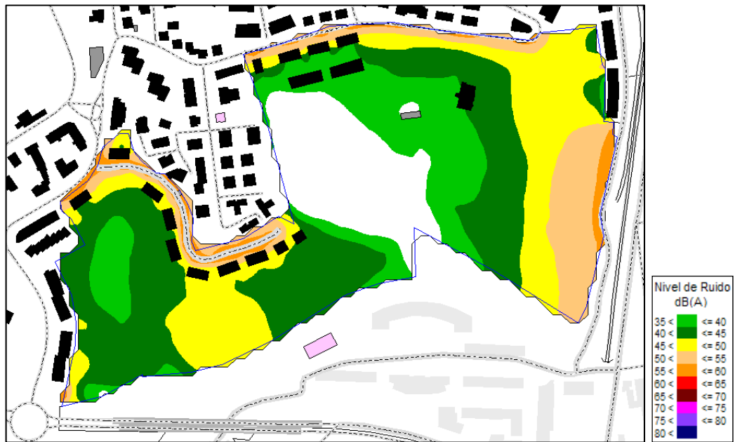
Nivel de ruido obtenido a 2m. de altura. Periodo noche
