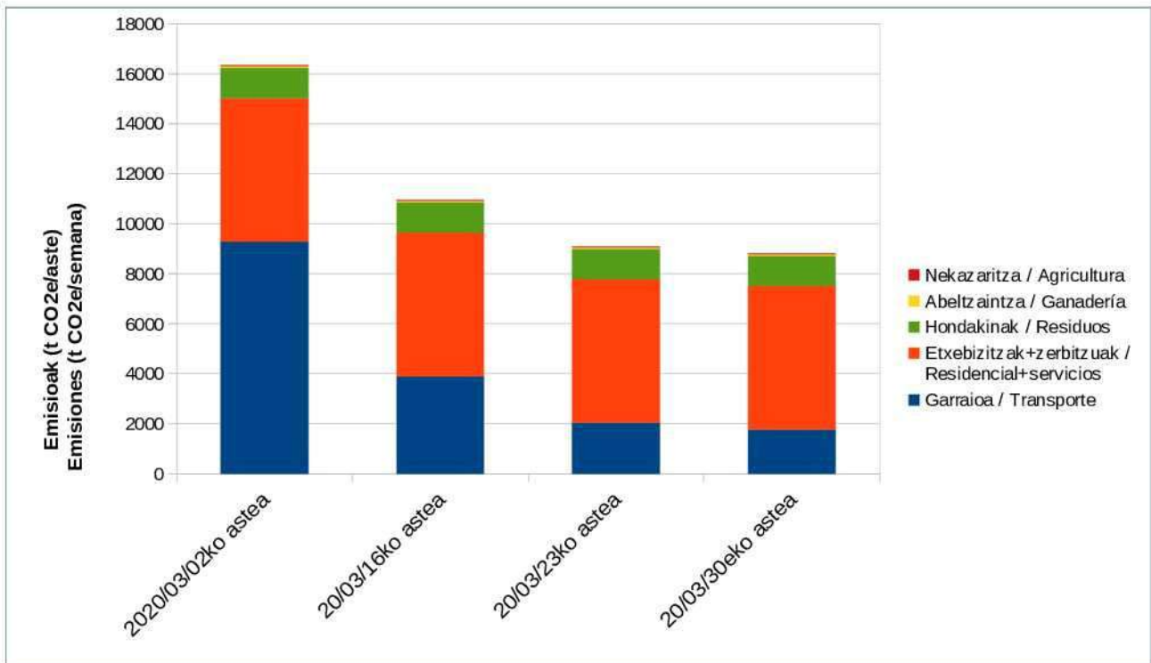
Gráfico 1. Simulación de las emisiones semanales de GEI durante las últimas semanas calculadas en función de los datos de tráfico en la ciudad y suponiendo que la suma de emisiones de los sectores residencial y servicios y que las emisiones de los residuos permanecen constantes.
