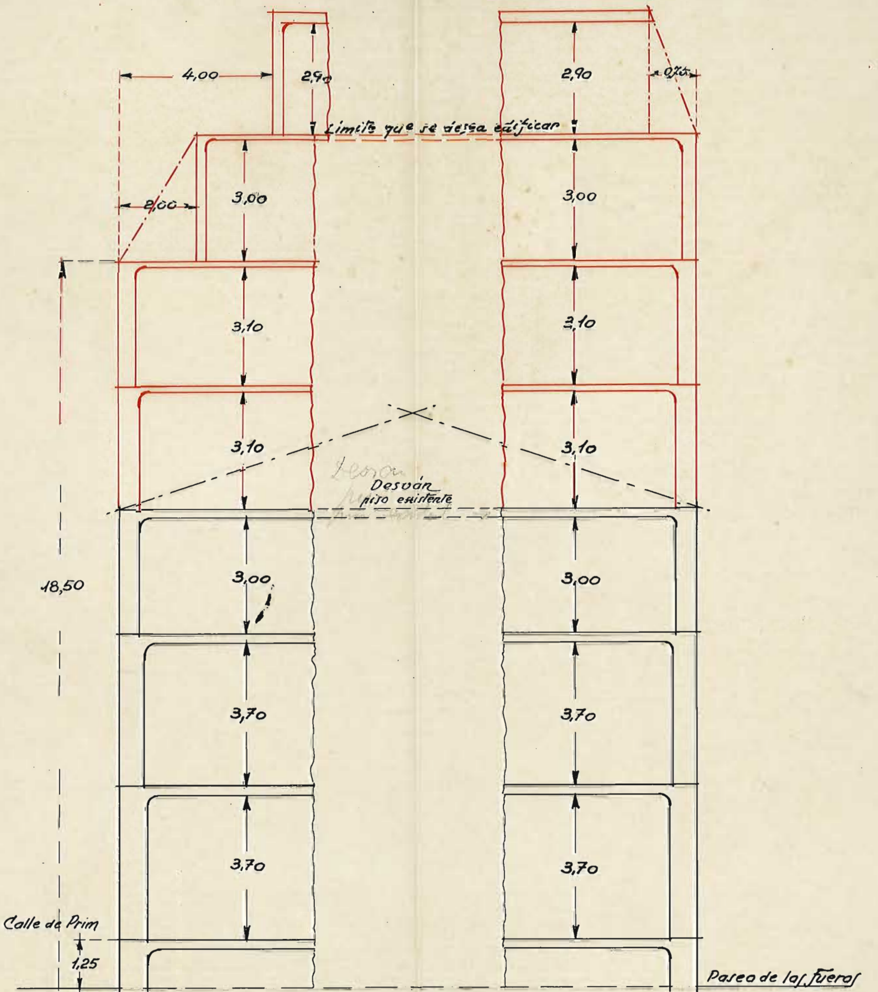
~ Perfil de 2º Orden ~
