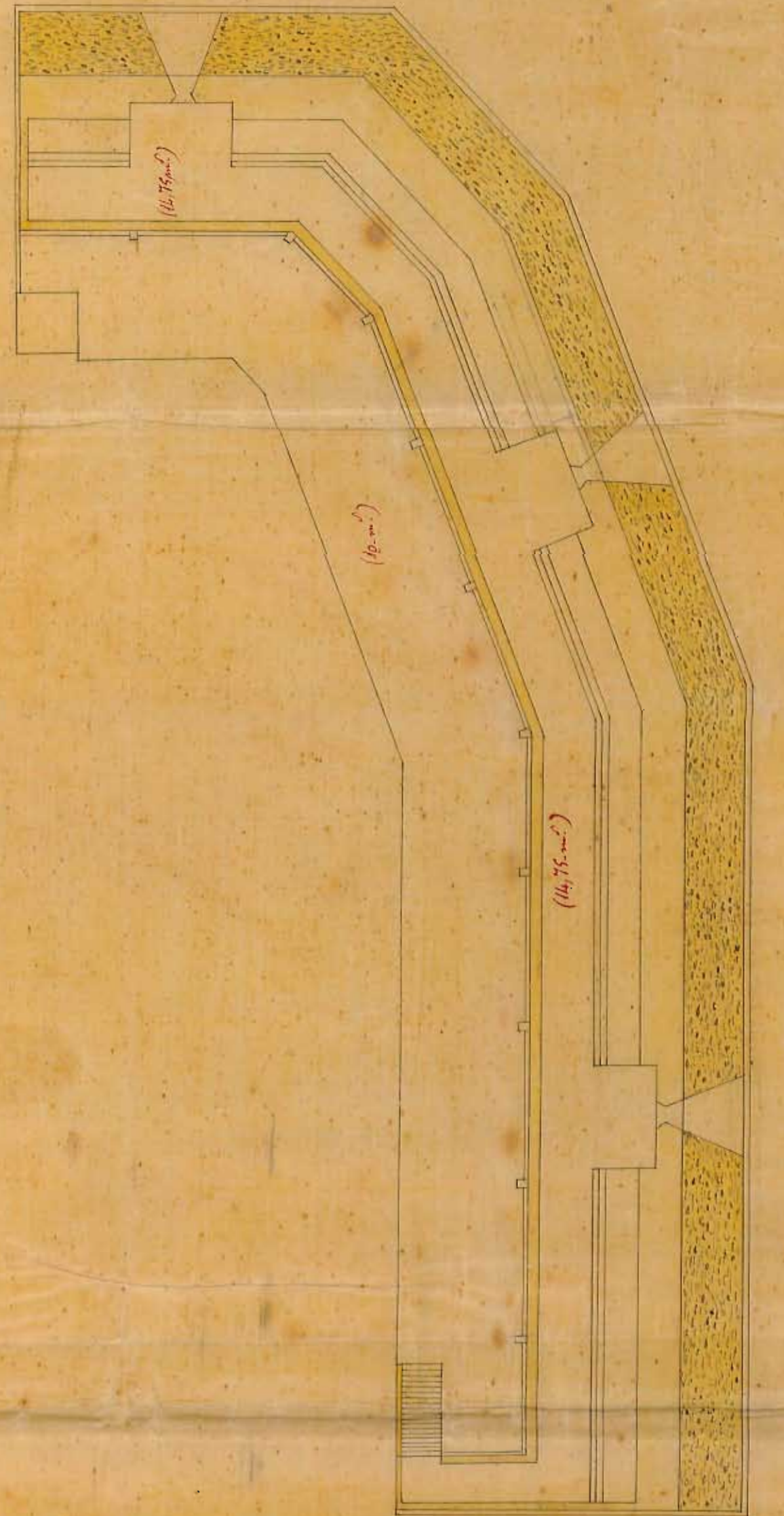
Plano del paso alto. Cuarta de N.
