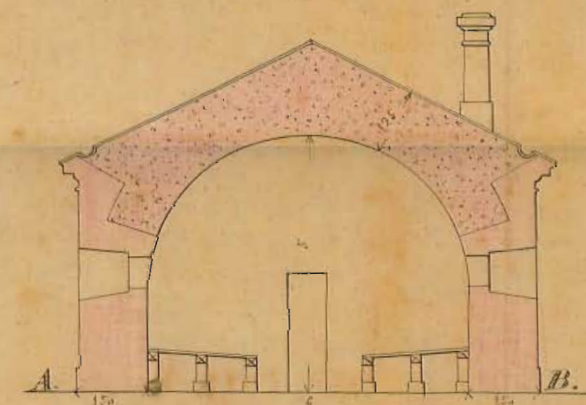
Perfil y vista por A.B.
