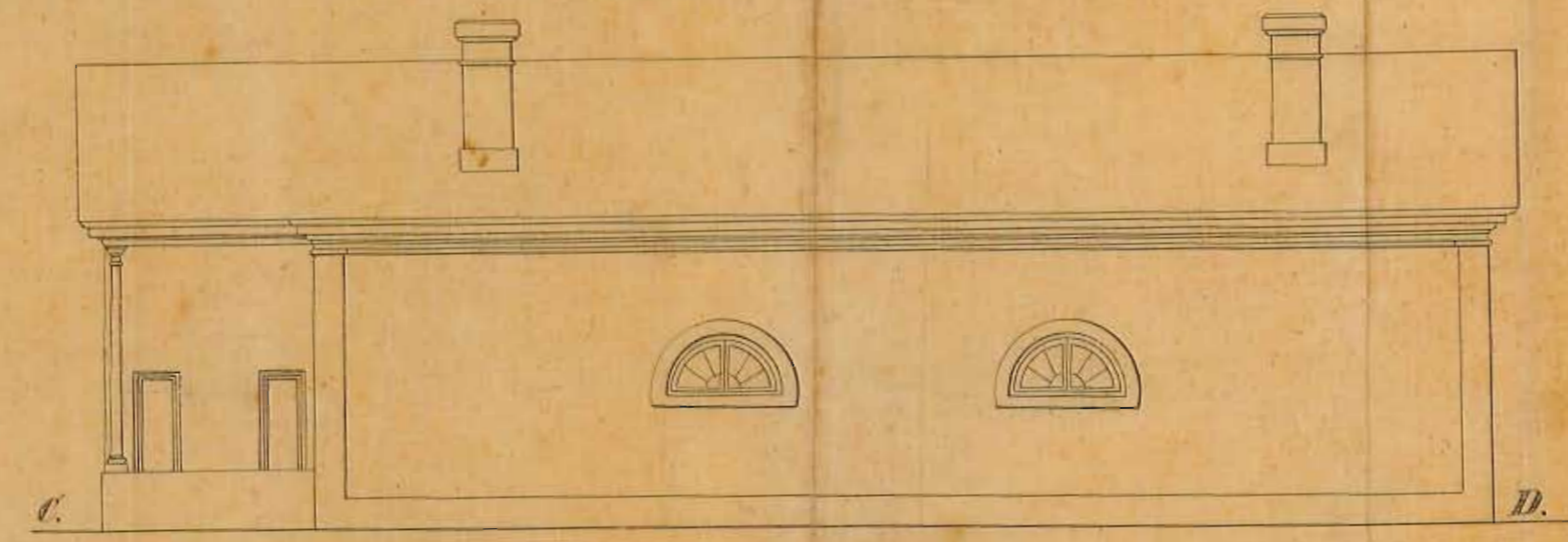
Alzado por C.D.
