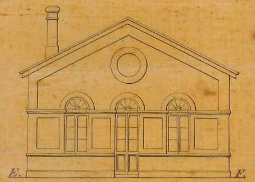
Alzado por E.F.
