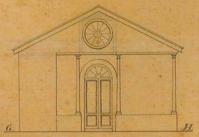
Alzado por G.H.
