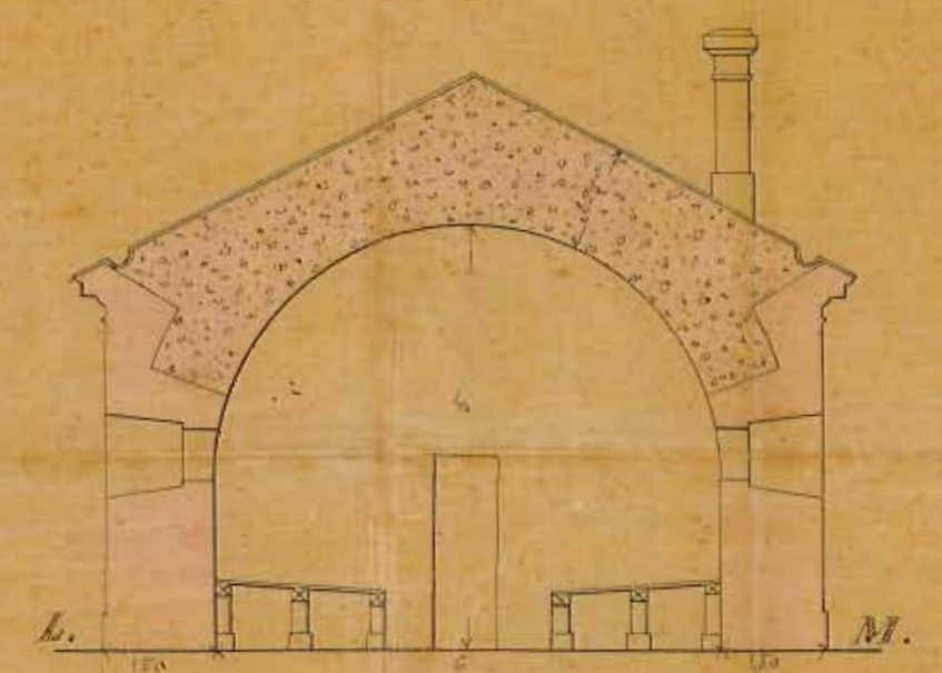
Perfil y vista por L.M.
