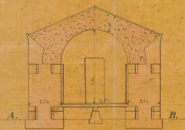
Perfil y vista por A.B.
