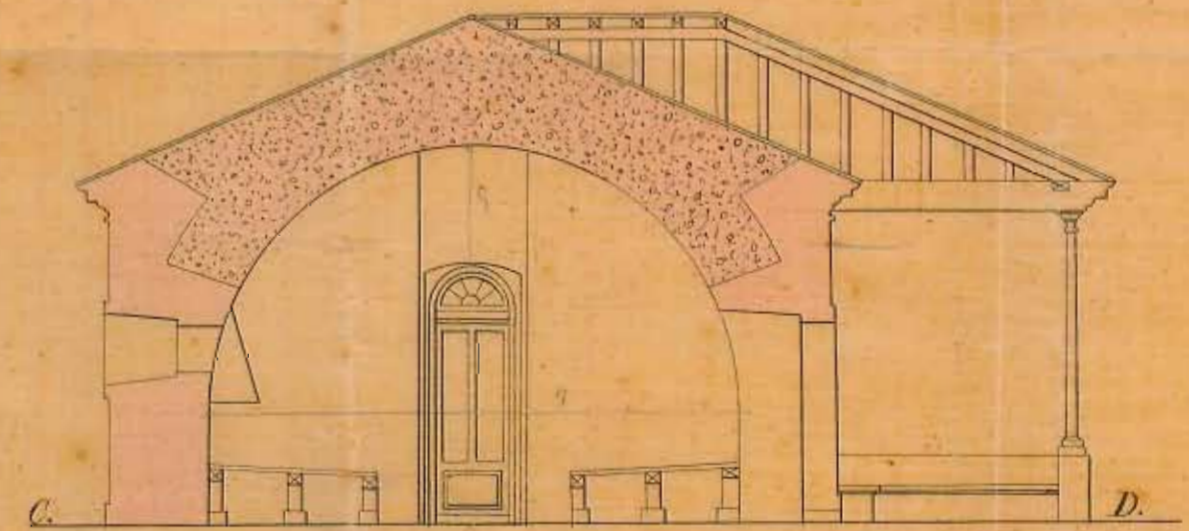
Perfil y vista por C. D.
