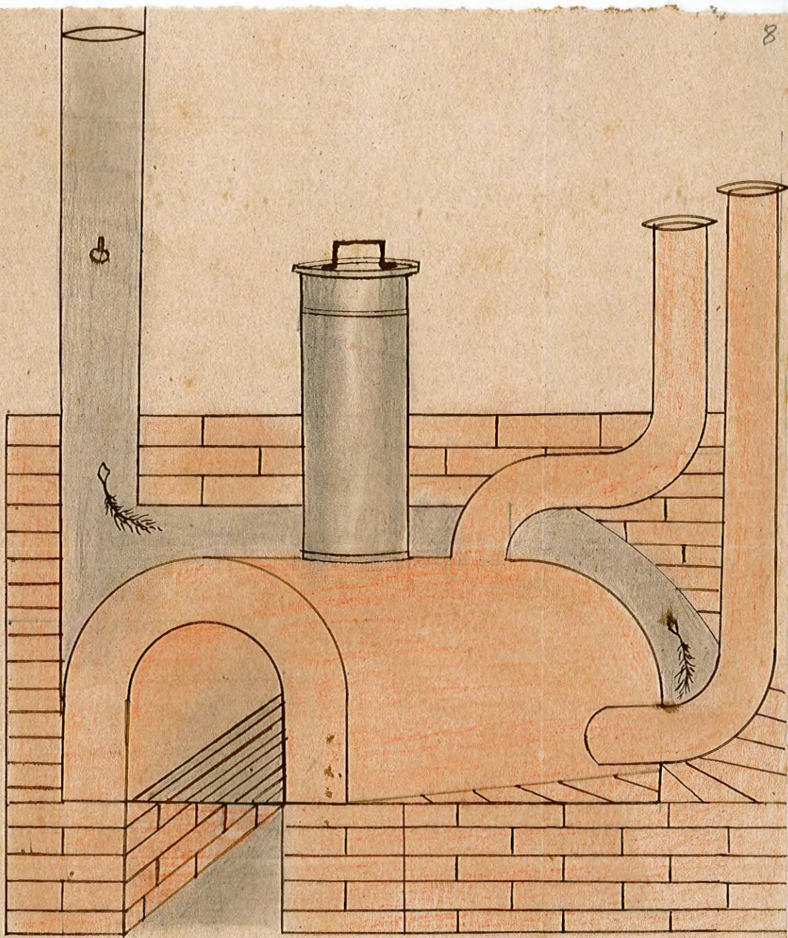
plan de chaudière et intérieur (dimension 0.60x0.30x0.12)
