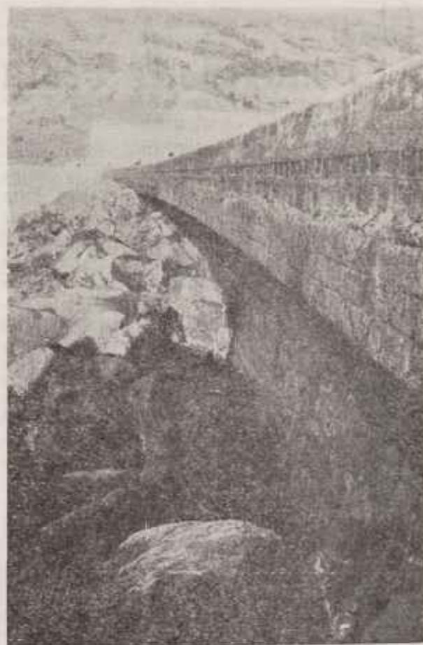
Muro de costa del Kursaal, después del temporal de 1965. Allí donde los bloques eran menos pesados, se notó un leve descenso en la escollera. Pero la obra y el muro resistieron perfectamente.
