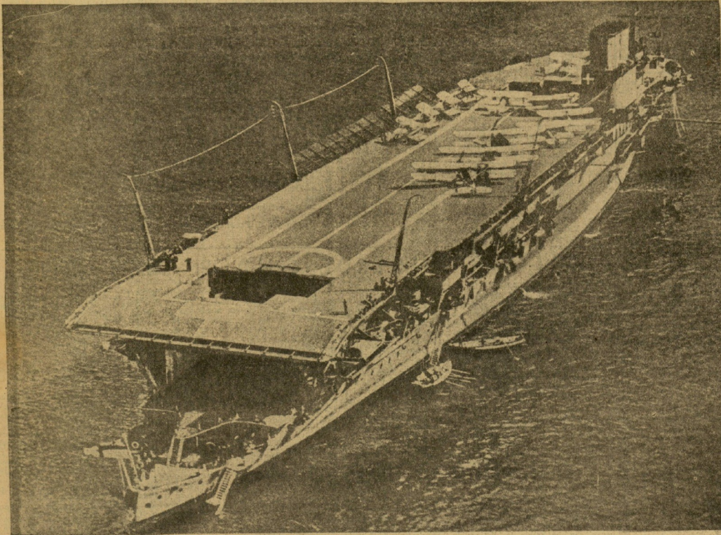
La ampliísima pista de aterrizaje y despegue de uno de los gigantescos portaaviones ingleses.
