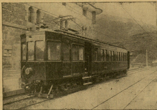
COCHE AUTOMOTOR DE VIAJEROS DEL FERROCARRIL DEL UROLA.
