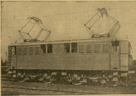
LOCOMOTORA ELECTRICA DE 1.500 HP. A 1.500 VOLTIOS.
