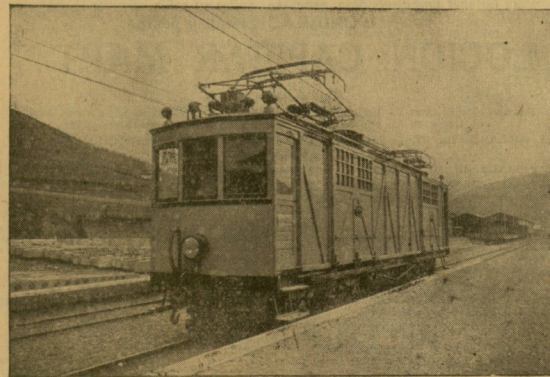
FURGON AUTOMOTOR DEL FERROCARRIL DEL UROLA.
