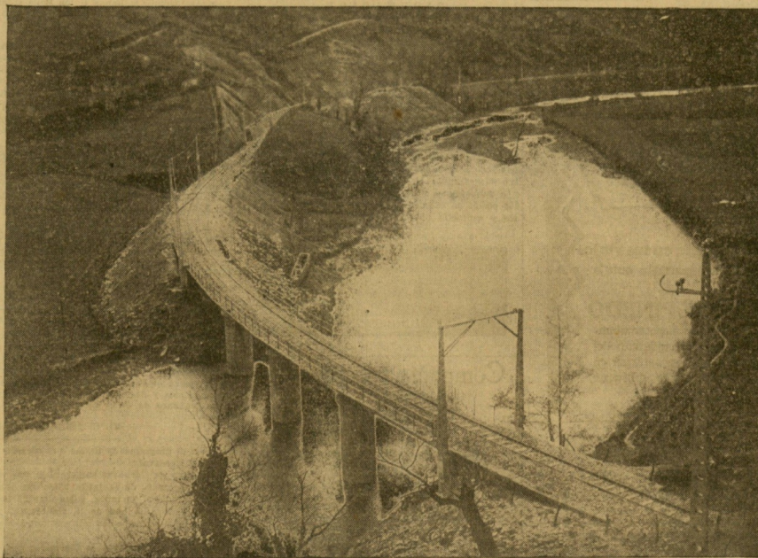
El puente de Badilegui, donde empezaron las obras del Urola: cuatro tramos de hormigón armado de 10'40 metros de luz.
