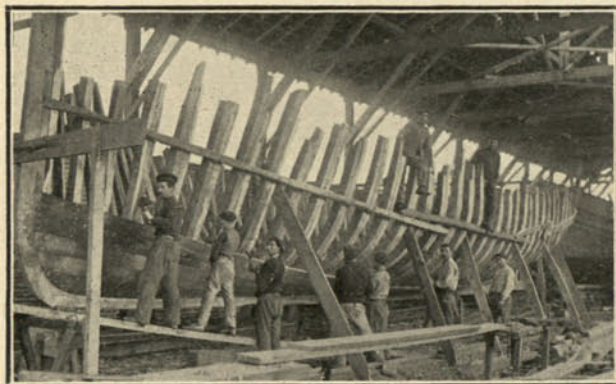
Vista interior de los Astilleros de D. Francisco Andonaegui, en Pasajes, y estado de construcción de algunos barcos.
