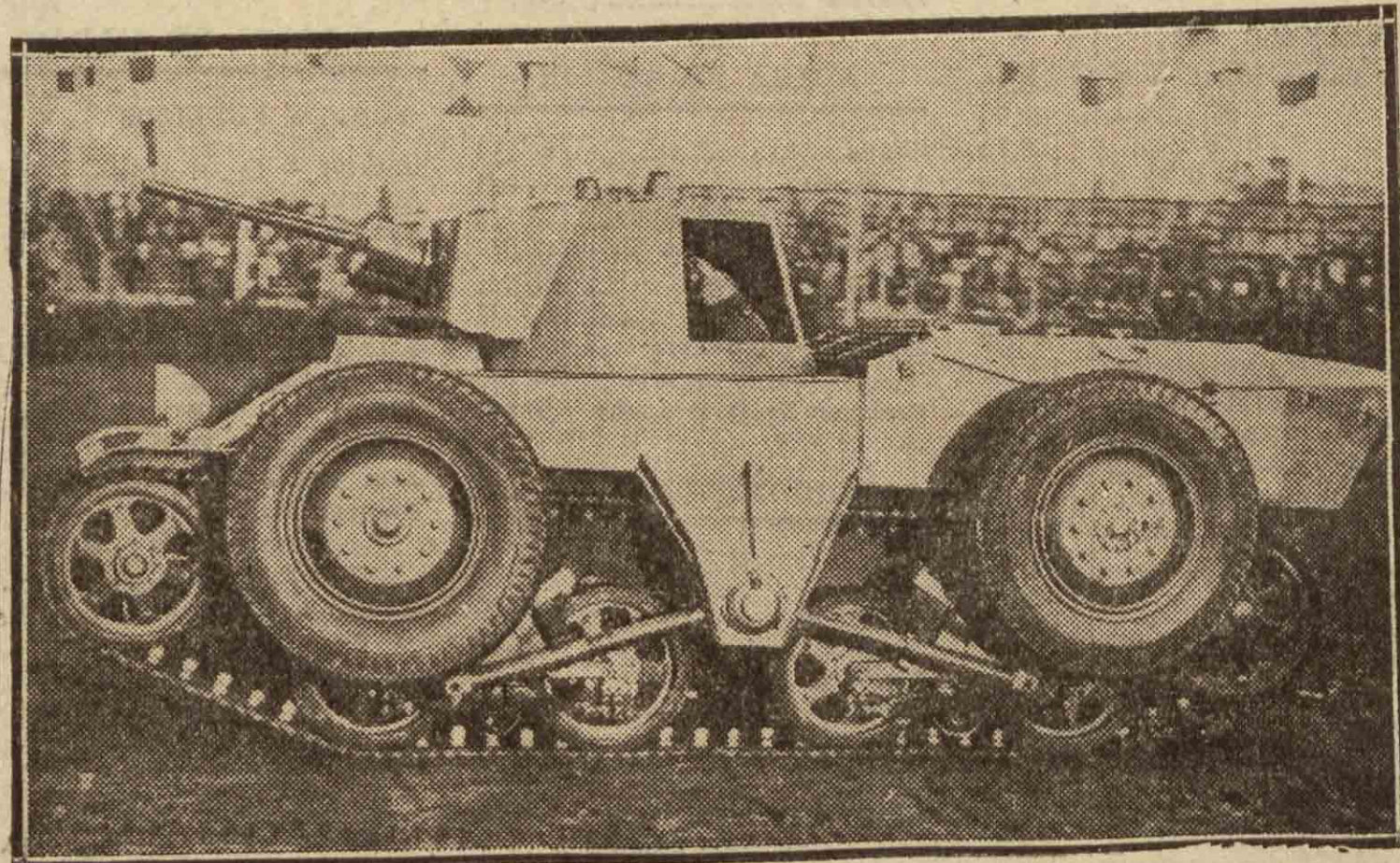
Es hueco; puede rodar tanto sobre el sistema «Oruga» como sobre ruedas. La velocidad sobre las orugas, es de 40 kilómetros por hora, y sobre las ruedas, de 75 km. Van tres hombres en el interior. Una ametralladora y un cañón, son su armamento.
