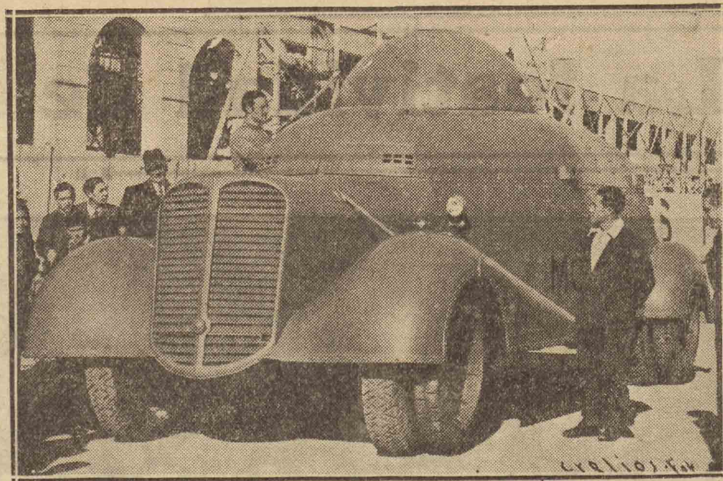
Nuevo modelo de automóvil blindado, construido totalmente en España, que ha sido adoptado por la Policía y la Guardia civil (Foto Contreras y Vilaseca.)
