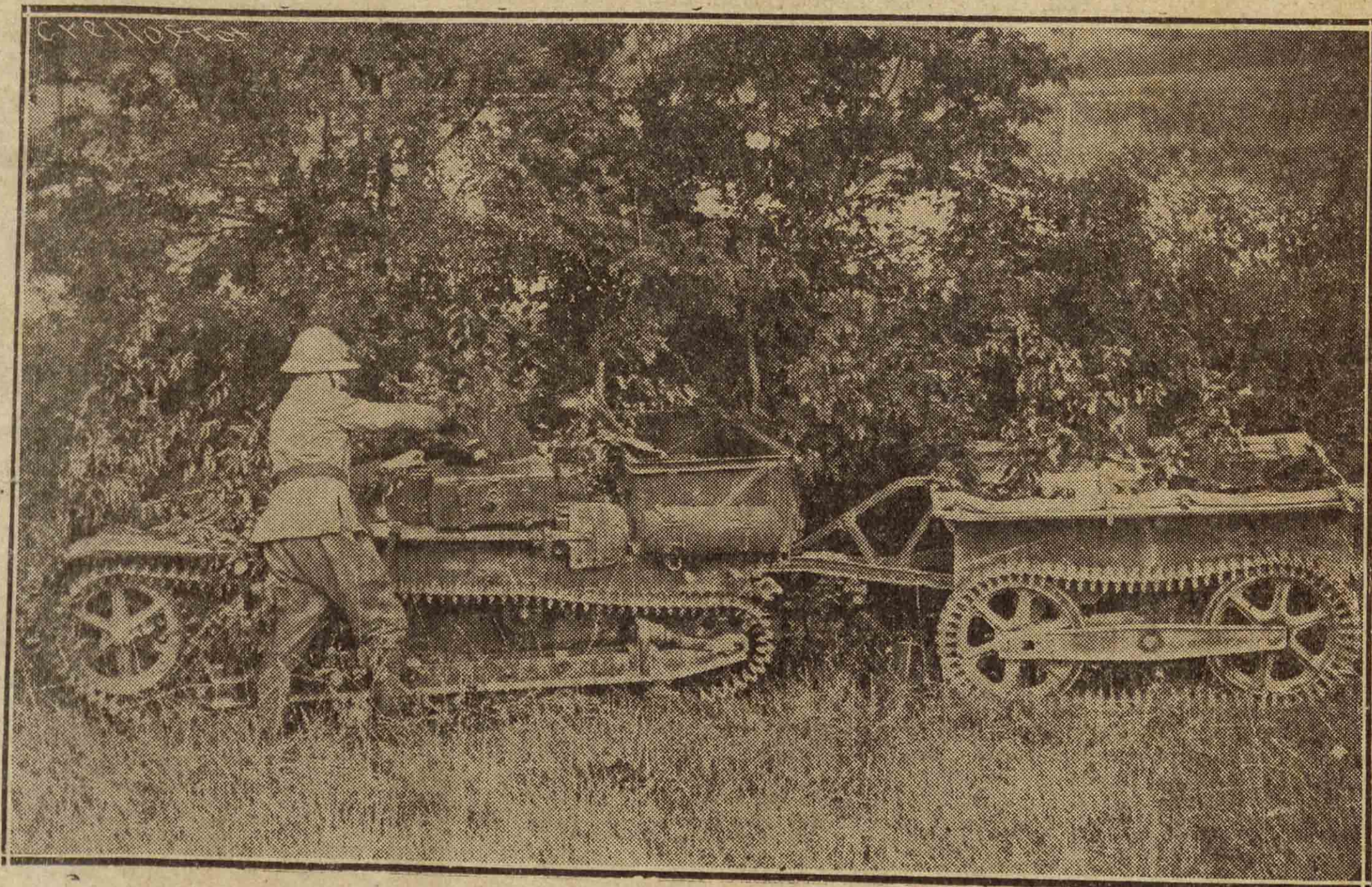
Carros rápidos, “orugas” que corren veloces por los campos. Ya no son aquellos tanques de la Gran Guerra. Estos de hoy son más perfectos. Así se ha demostrado en las grandes maniobras del campo de Mailly, en Francia. (Foto Gil del Espinar.)
