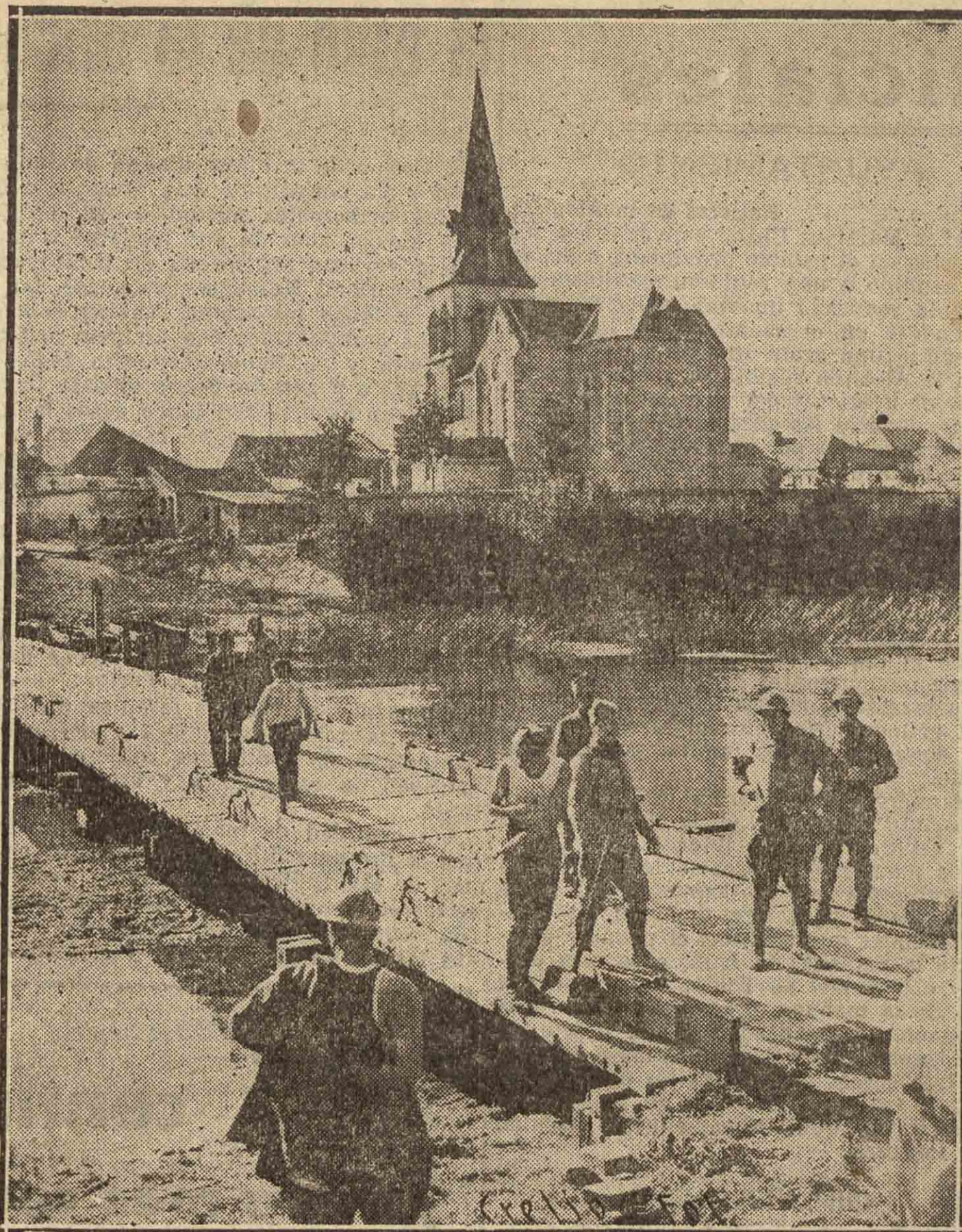
Los soldados de ingenieros franceses que están de maniobras en la región de Reims, tan tendido un puente sobre el río Marne
