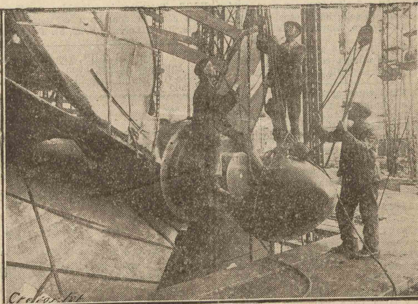
Mejor idea podrá hacerse de las dimensiones de "Cunarder 534" a la vista de las paletas de una de las enormes hélices cuyo montaje están terminando estos obreros, uno de los cuales está montado sobre la tuerca gigantesca cuyo tapón preparan (Foto Hernando.)
