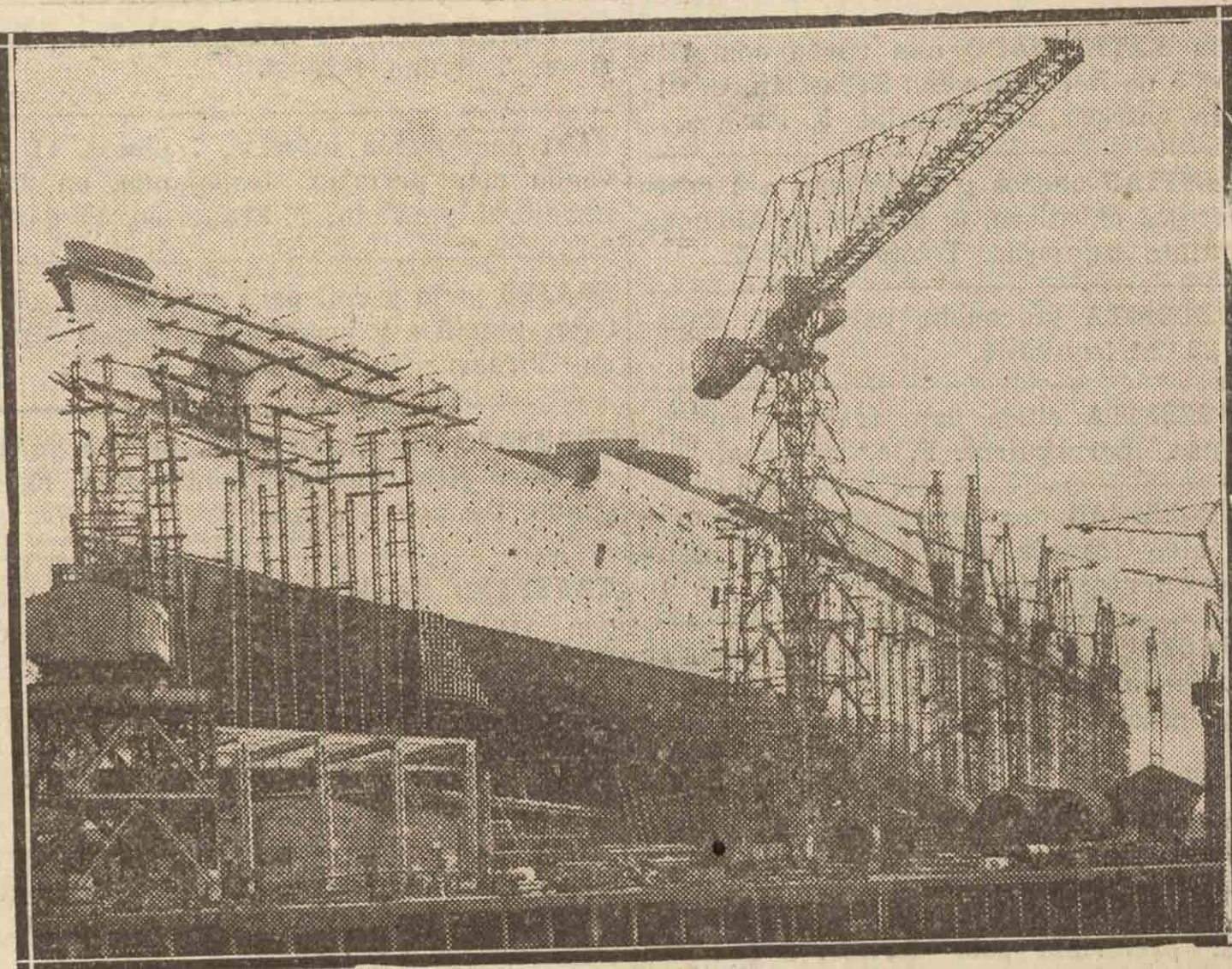
El día 26 del mes en que entramos hoy será botado al agua el gigante "Cunarder 534", nuevo paquebote que será el mayor del mundo. En la foto, tomando como punto de comparación los tanques y las grúas gigantes, puede hacerse idea de las dimensiones del buque.
