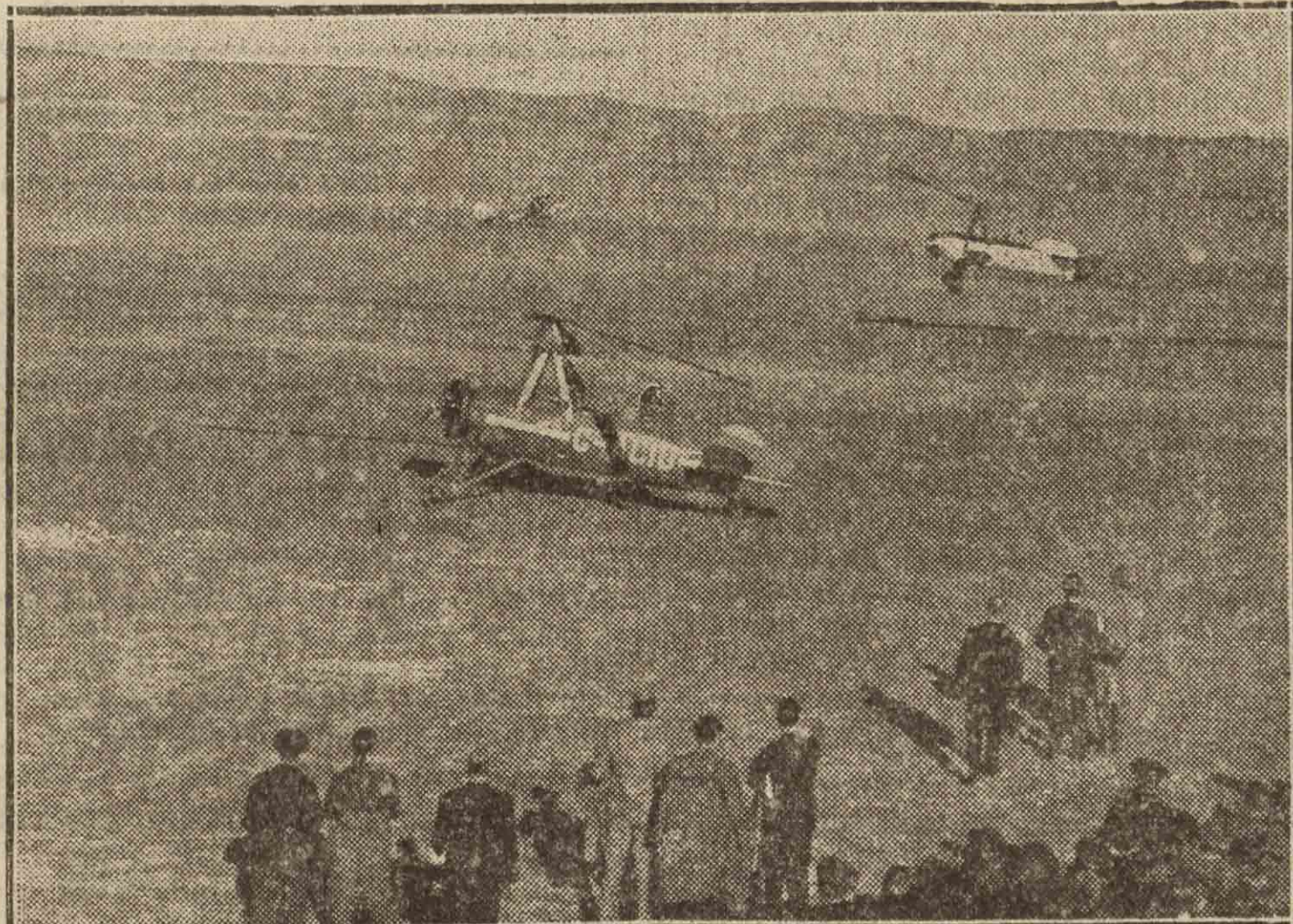
MADRID. — He aquí un momento de la brillante fiesta de aviación celebrada en homenaje al ingeniero español don Juan de la Cierva. El antiguo modelo de autogiro acaba de tomar tierra. Y el nuevo modelo va a aterrizar en el reducidísimo espacio que necesita. (Foto Contreras y Vilaseca.)
