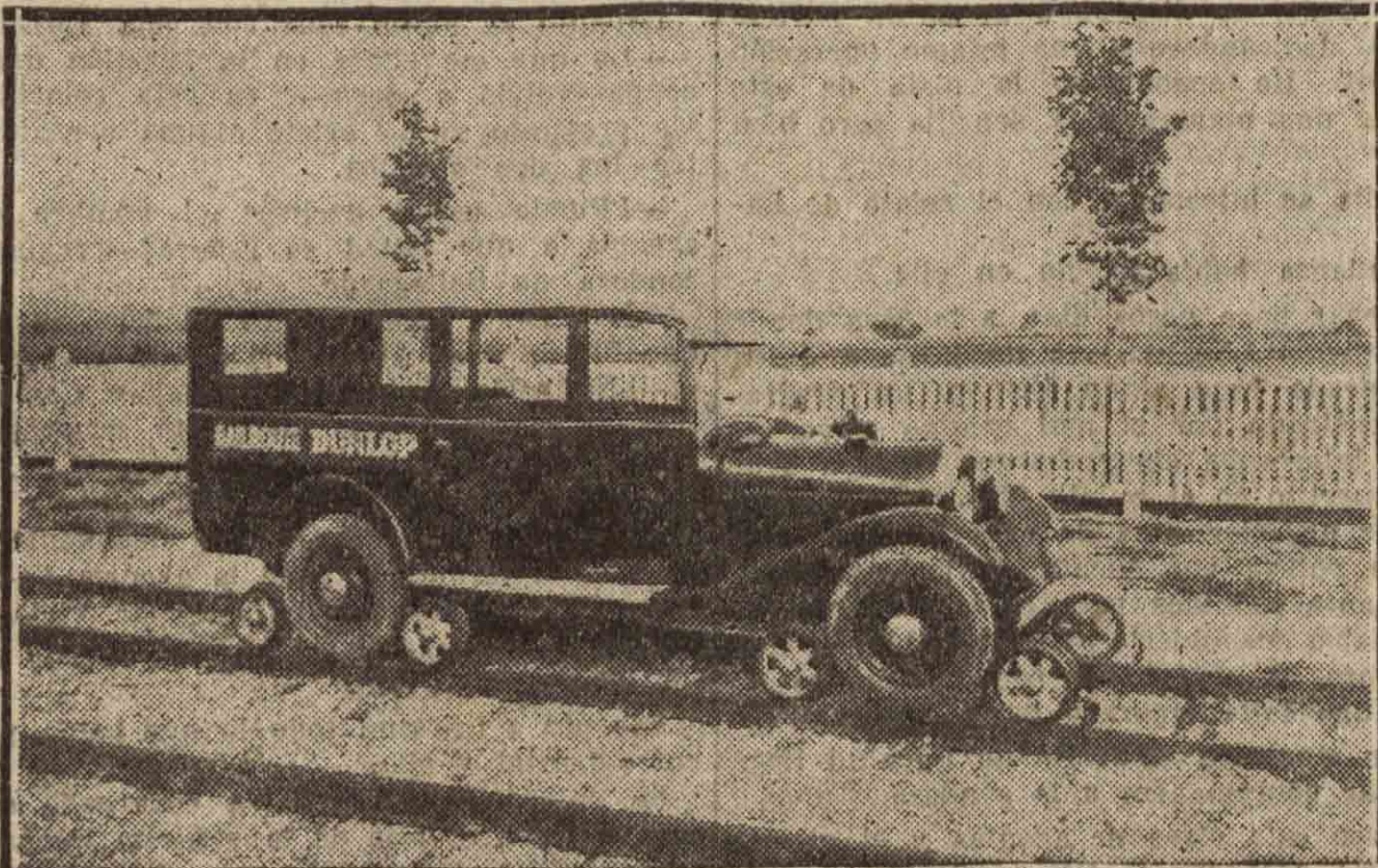
El auto "Railroute" sobre rail, experimentado felizmente en la nueva línea férrea de Gannat a la Fertee-Hautrive, en presencia del ministro de Obras Públicas francés y de los ingenieros de ferrocarriles (Foto Rol.)
