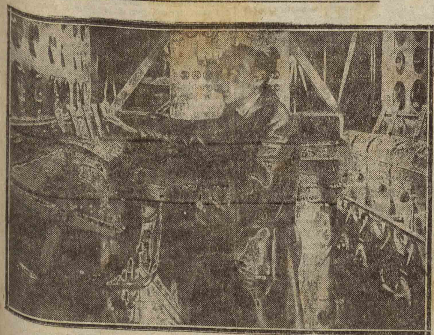
Un aspecto de la cabina de mando del gran hidroplano de 12 motores «DO-X», construido por Dornier. (Foto Consorcio.)
