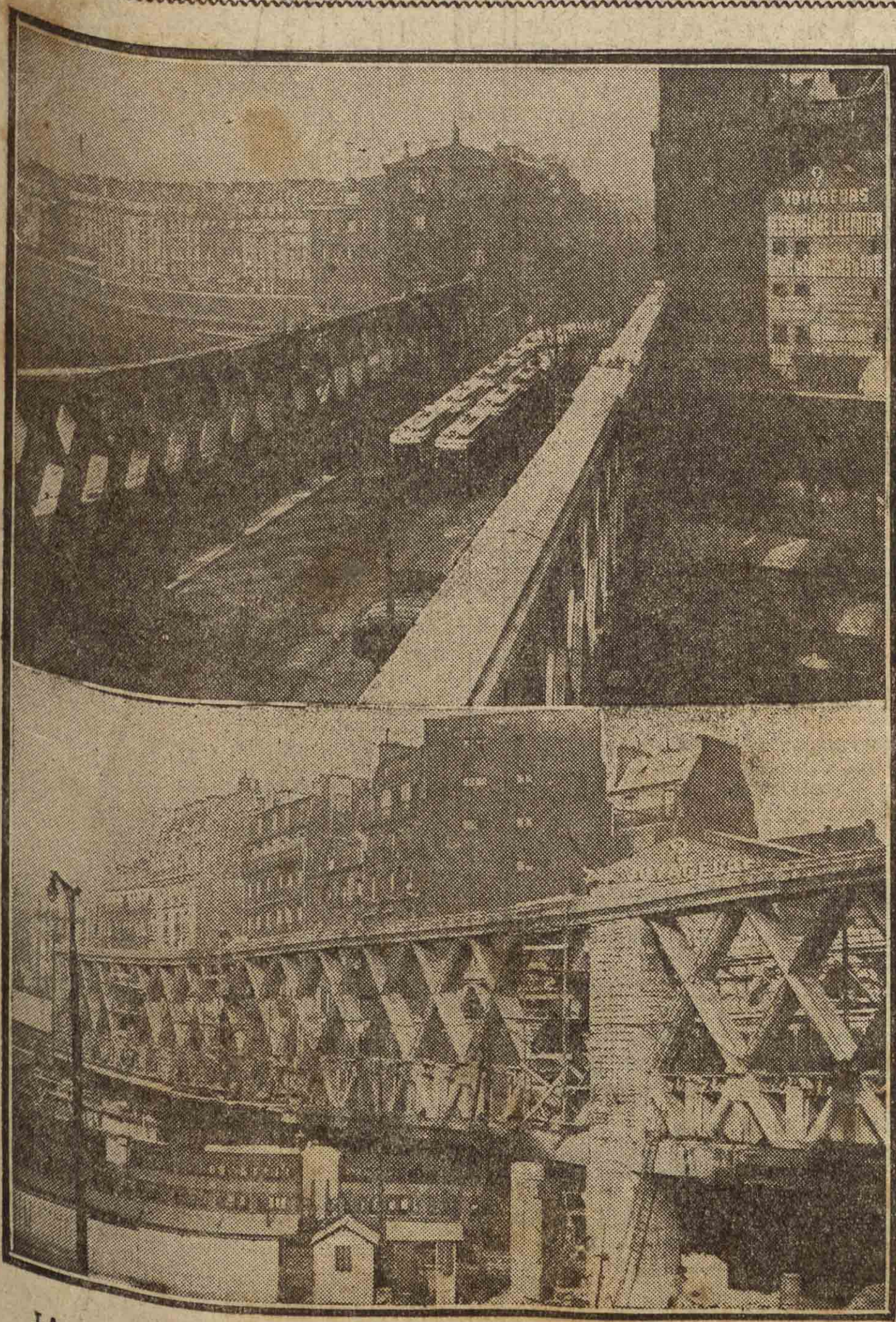
LA ACTUALIDAD GRAFICA EXTRANJERA. — Arriba, ensayos de resistencia en el nuevo puente de cemento armado construido en París sobre la estación del Este; y, abajo, el nuevo puente, visto desde abajo. (Foto Consorcio.)
