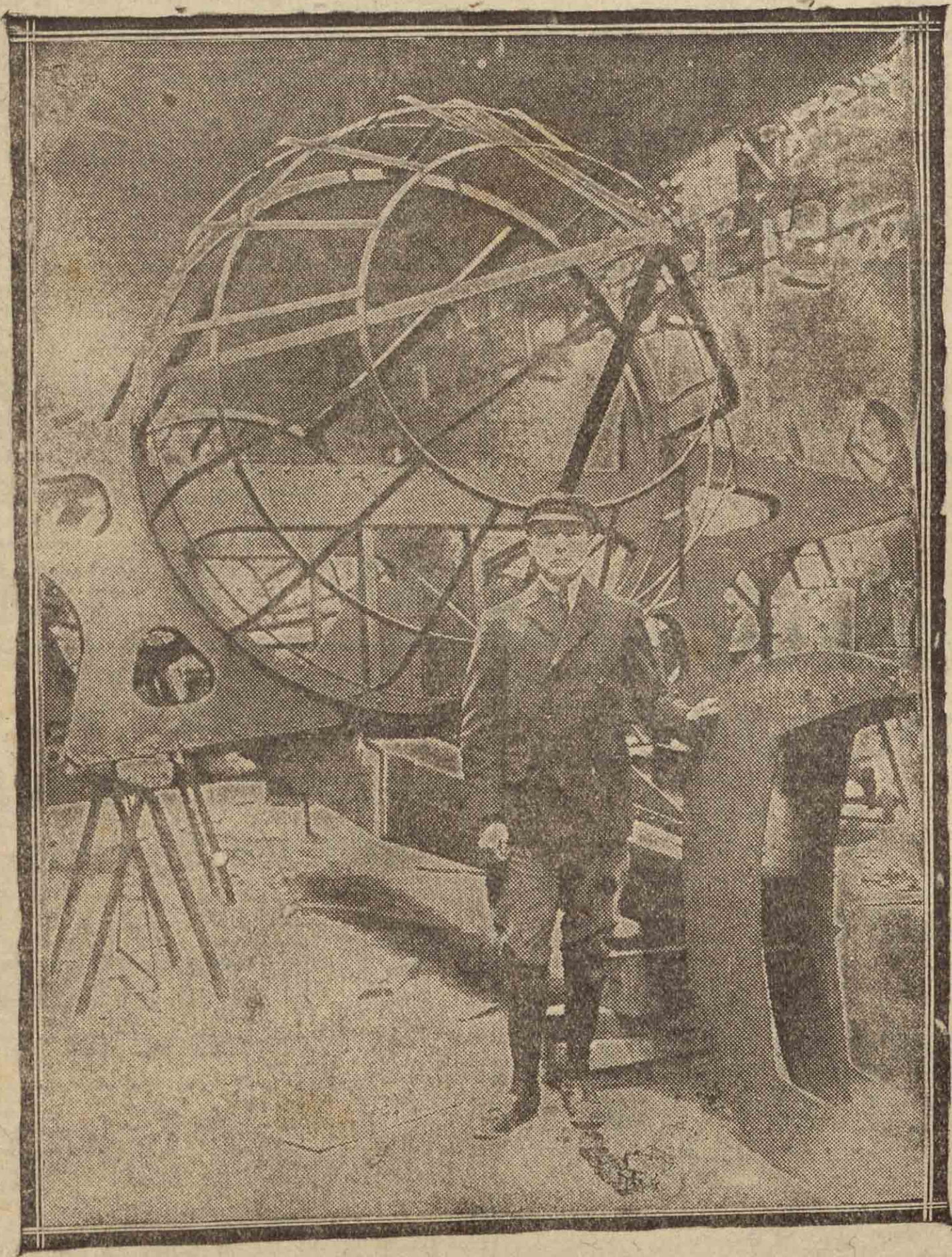
El aparato en el que el ingeniero Reony Compte intentará la travesía aérea del Atlántico. La nueva máquina está a punto de terminarse, pesa nueve toneladas y consta de una cabina de nueve metros de largo por 2,50 m. de ancho. (Fot. Consorcio.)
