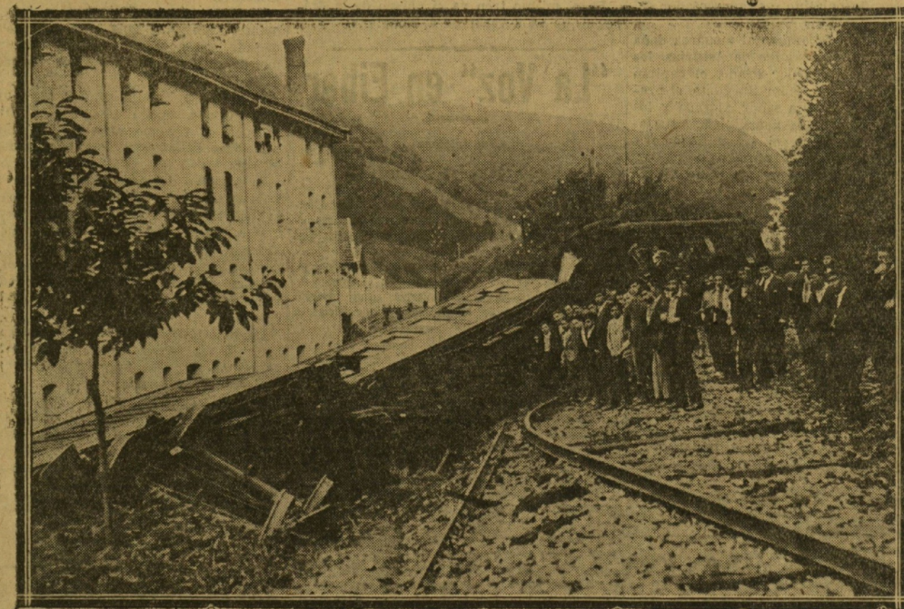
Estado en que quedaron los dos vagones volcados y los carriles destrozados a causa del accidente.
