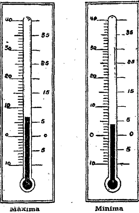
SITUACION ATMOSFERICA
