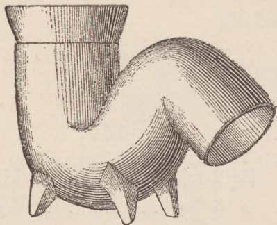
Sifón de patas.
