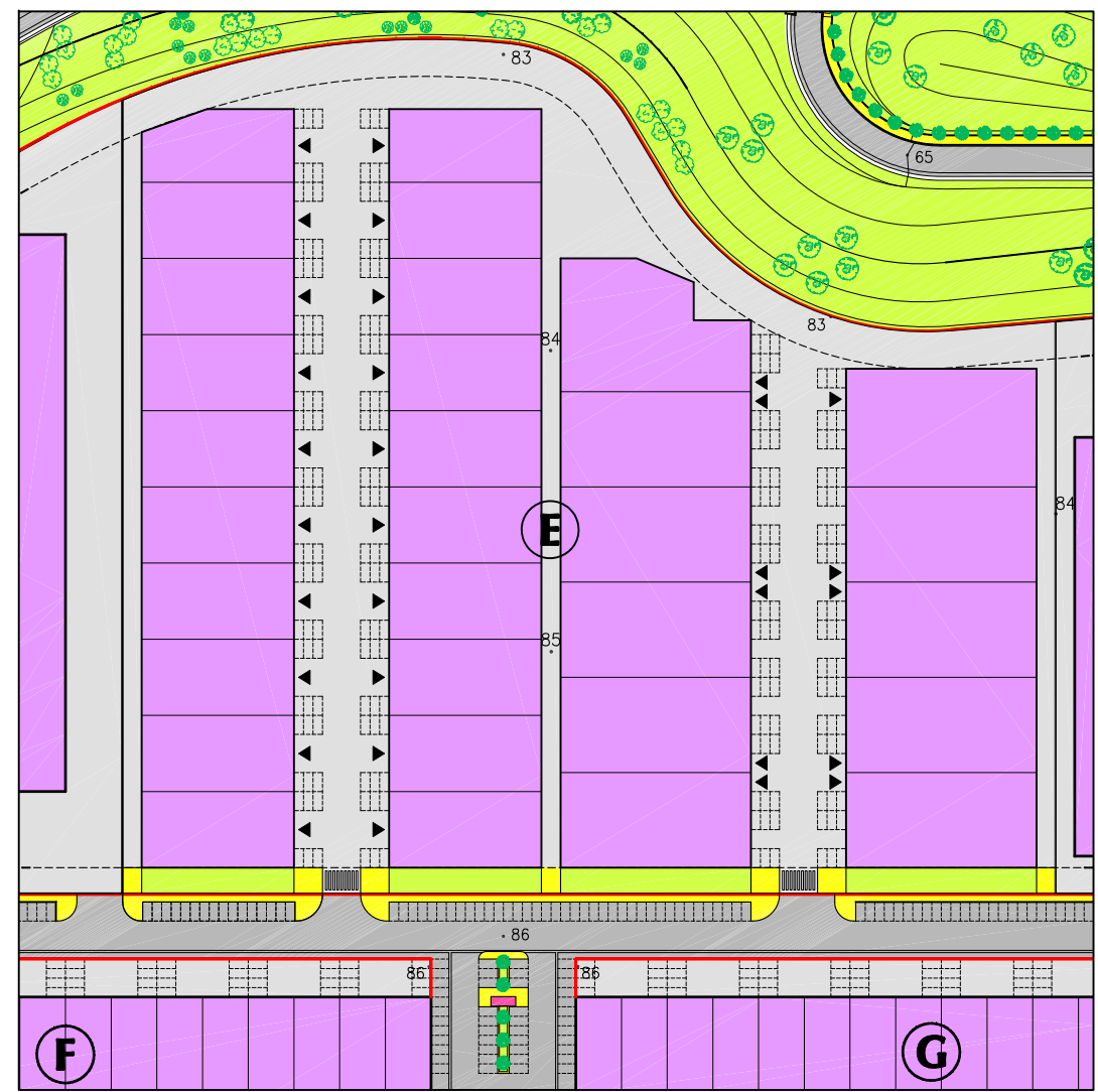
ALTERNATIVA DE ORDENACION TIPOLOGICA EN PARCELA "E"
