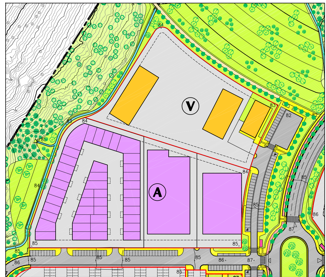
ALTERNATIVA DE ORDENACION TIPOLOGICA EN PARCELA "A"
