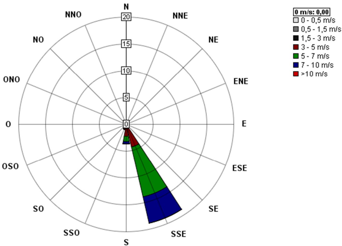
Gráfica 3. Rosa de los vientos (19 de diciembre)
