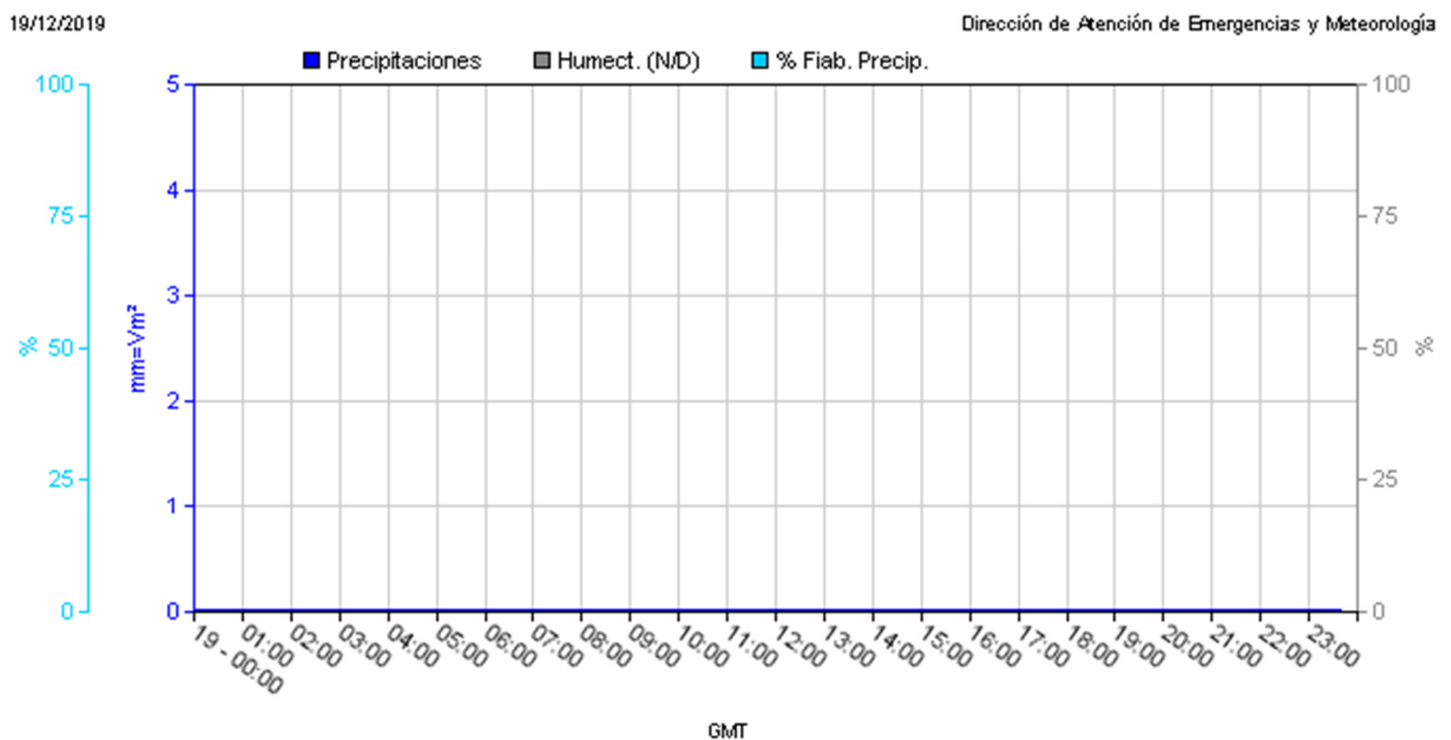
Gráfica 2. Perfil de pluviometría (19 de diciembre)
