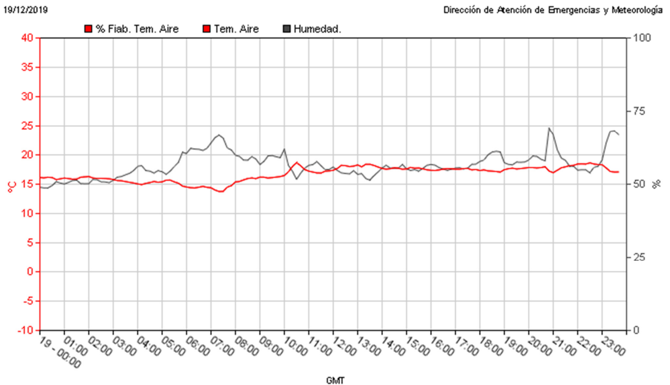
Gráfica 1. Perfil de temperatura y humedad (19 de diciembre)
